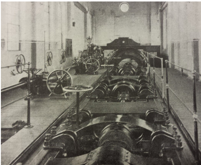
Wasserkraftanlage Berka/Werra 1909
