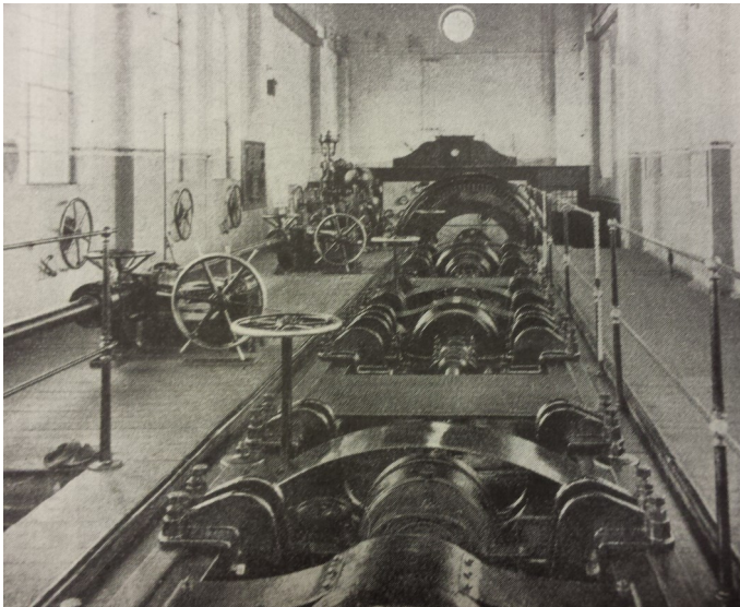
Wasserkraftanlage Berka/Werra 1909
