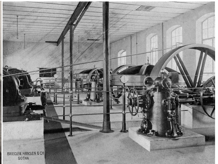
Überlandzentrale Mihla/Werra 1910
